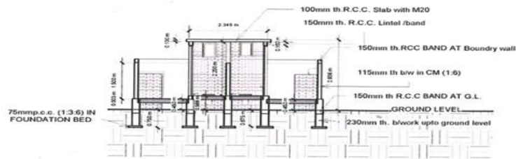
③ Section 1 1 : 96
