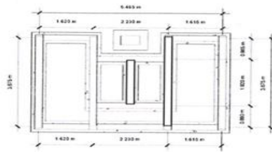
④ foundation 1 : 96
